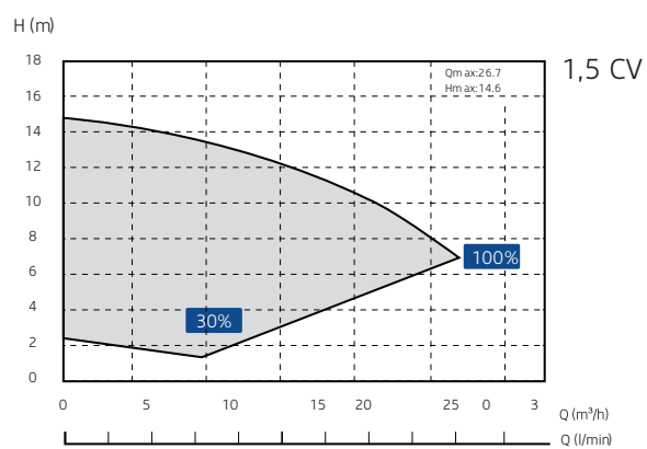
Curva de desempenho - 1 CV • 1,5 CV
