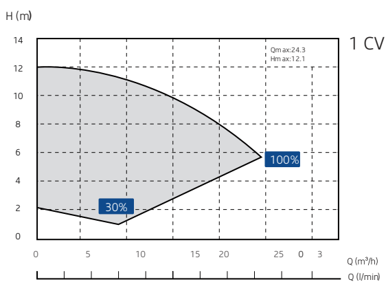
Curva de desempenho - 1 CV • 1,5 CV
