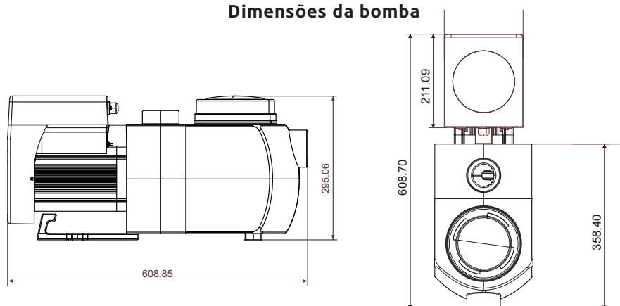
Dimensões da bomba
